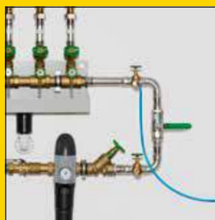
Druktest met perslucht (SL/SLW)
